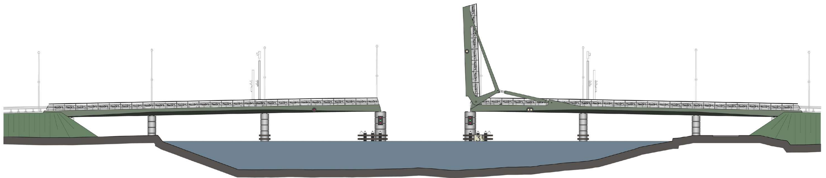
zij aanzicht brug open
