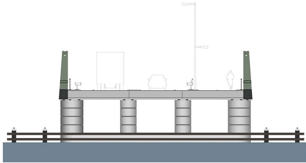
dwarsdoorsnede brug t.p.v. het val
