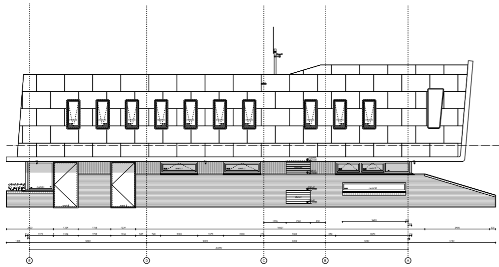
Noordgevel
