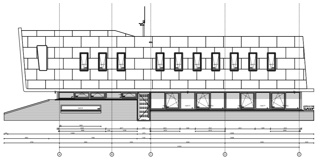
Zuidgevel
