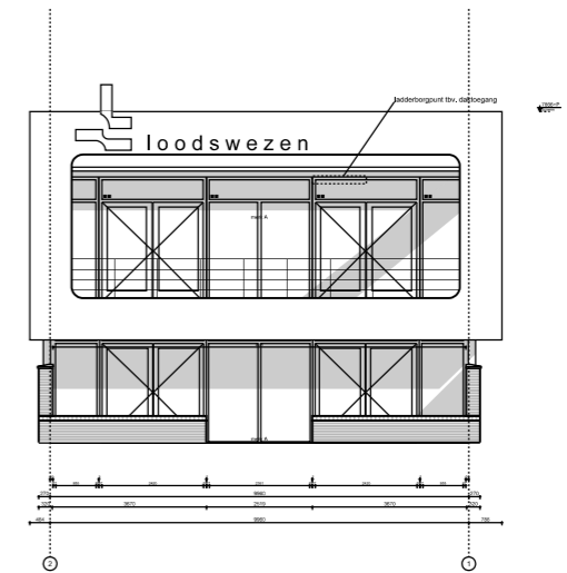
Westgevel
