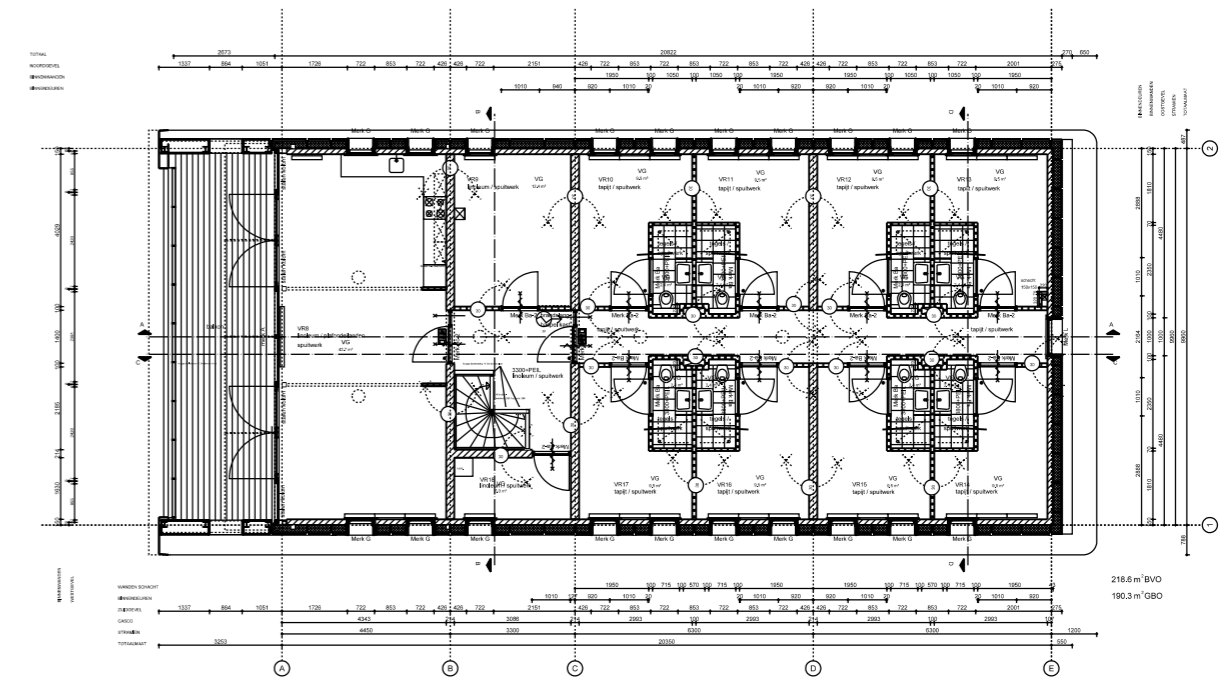
Begane grond 1 : 200
