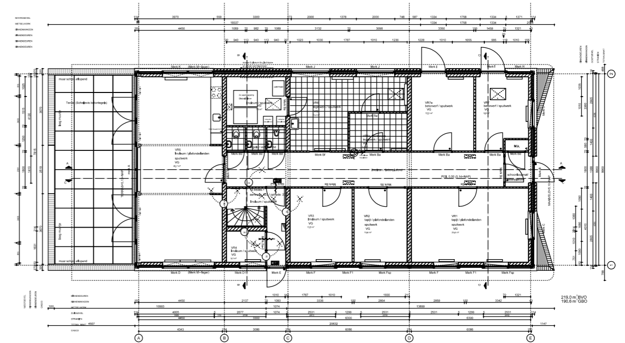
Eerste verdieping 1 : 200
