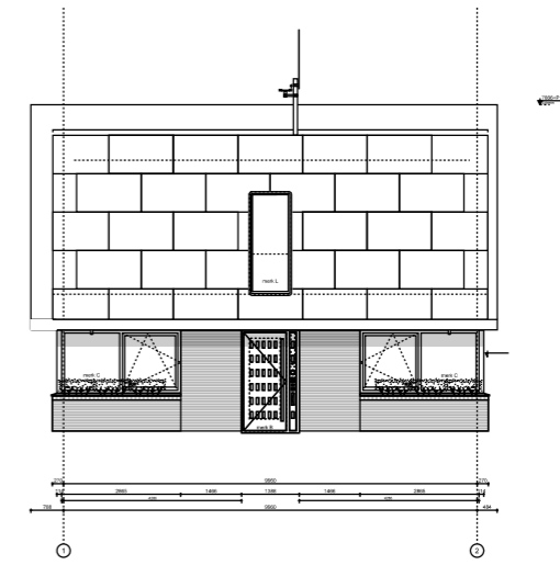
Noordgevel
