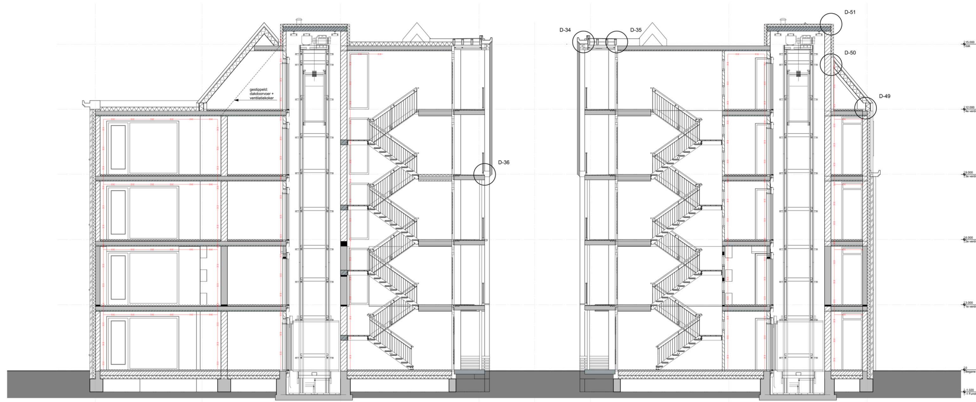
doorsnede CC
