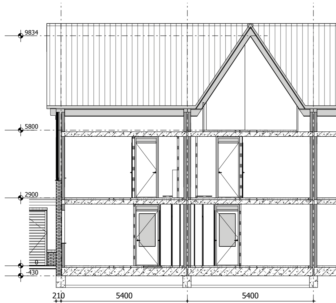
Doorsnede
