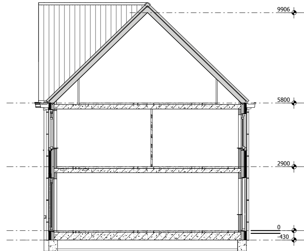
Doorsnede
