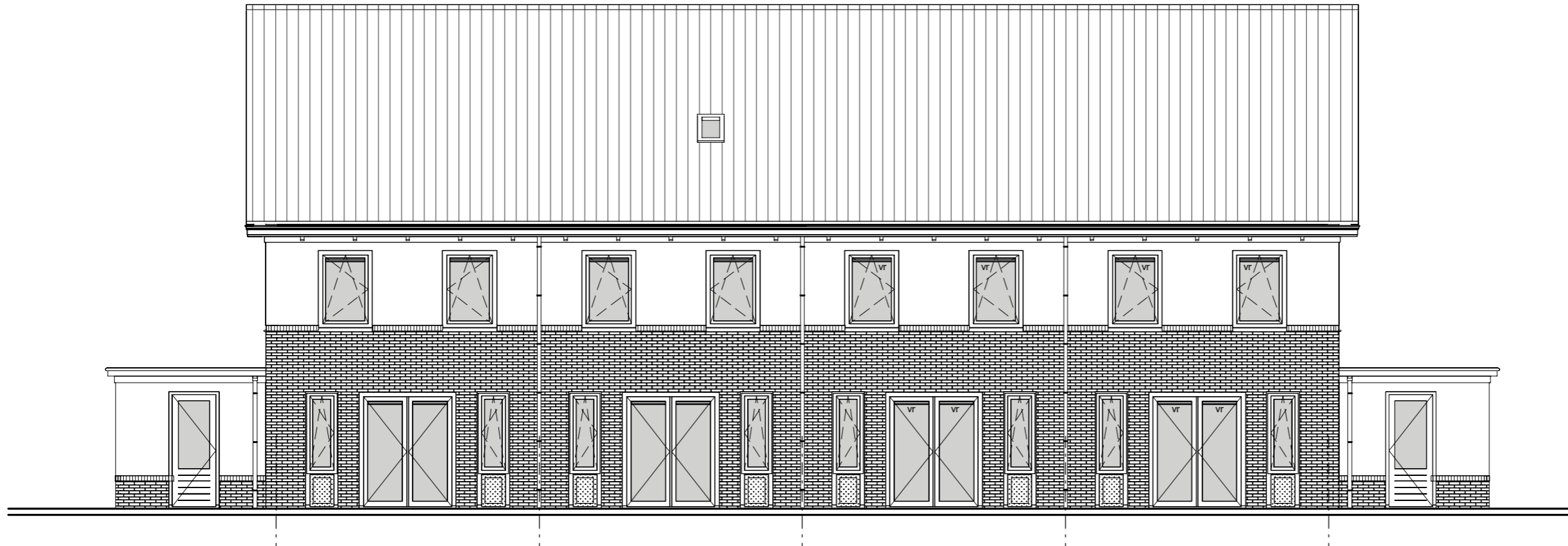
Achtergevel
