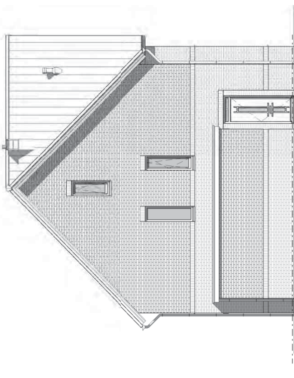
Linker zijgevel
