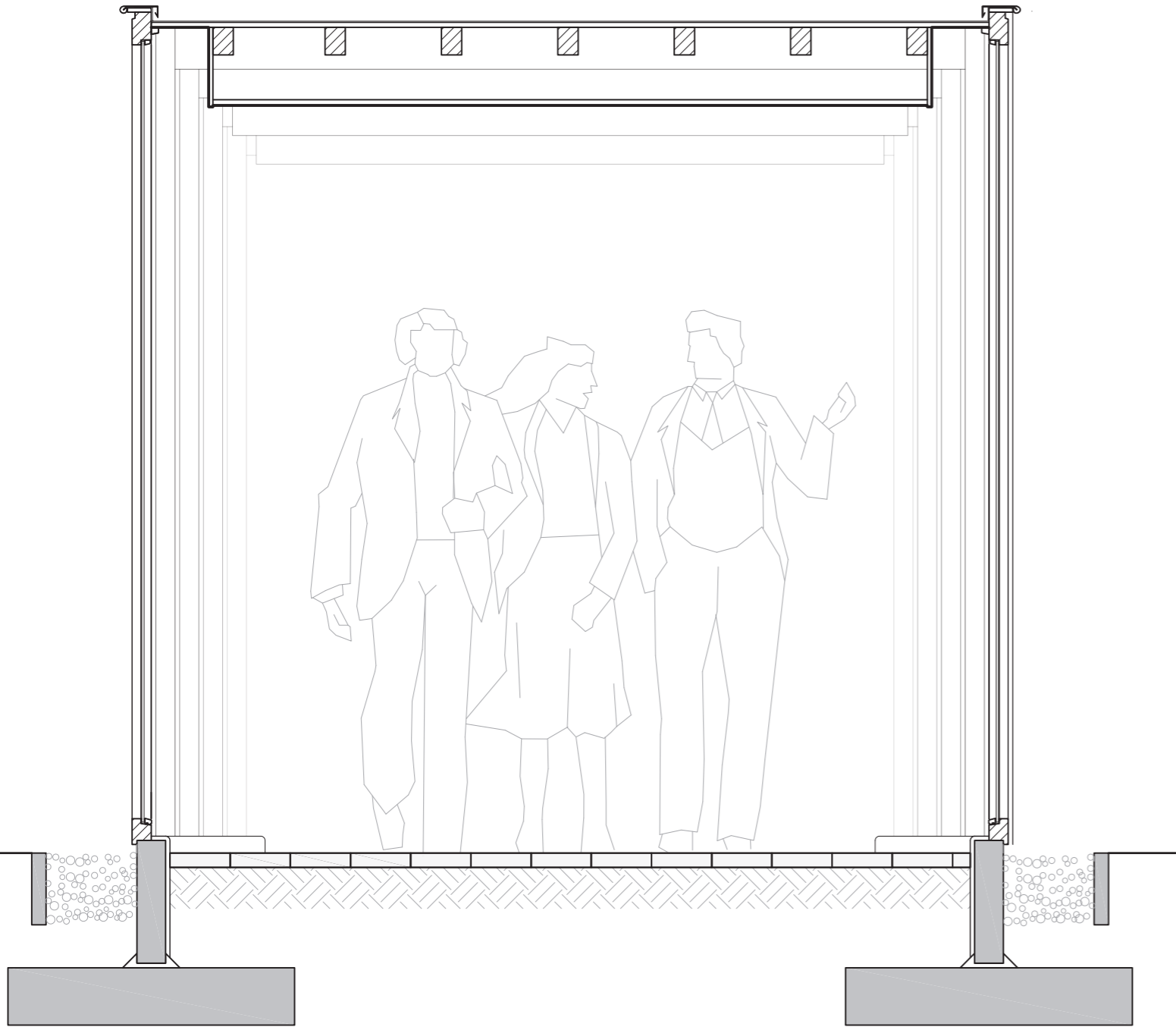
Dwarsdoorsnede corridor
