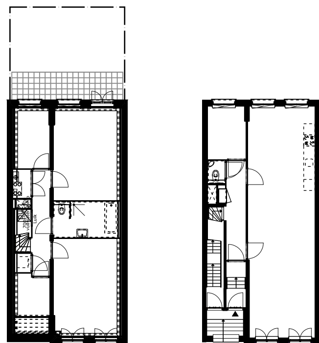
Souterrain
