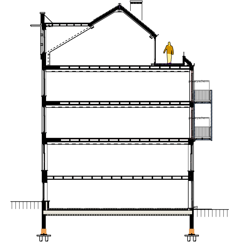
Doorsnede
