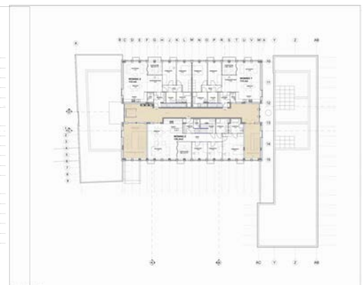
Noordblok PG 2 e verdieping nieuw
