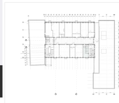
Noordblok PG 2 e verdieping bestaand
