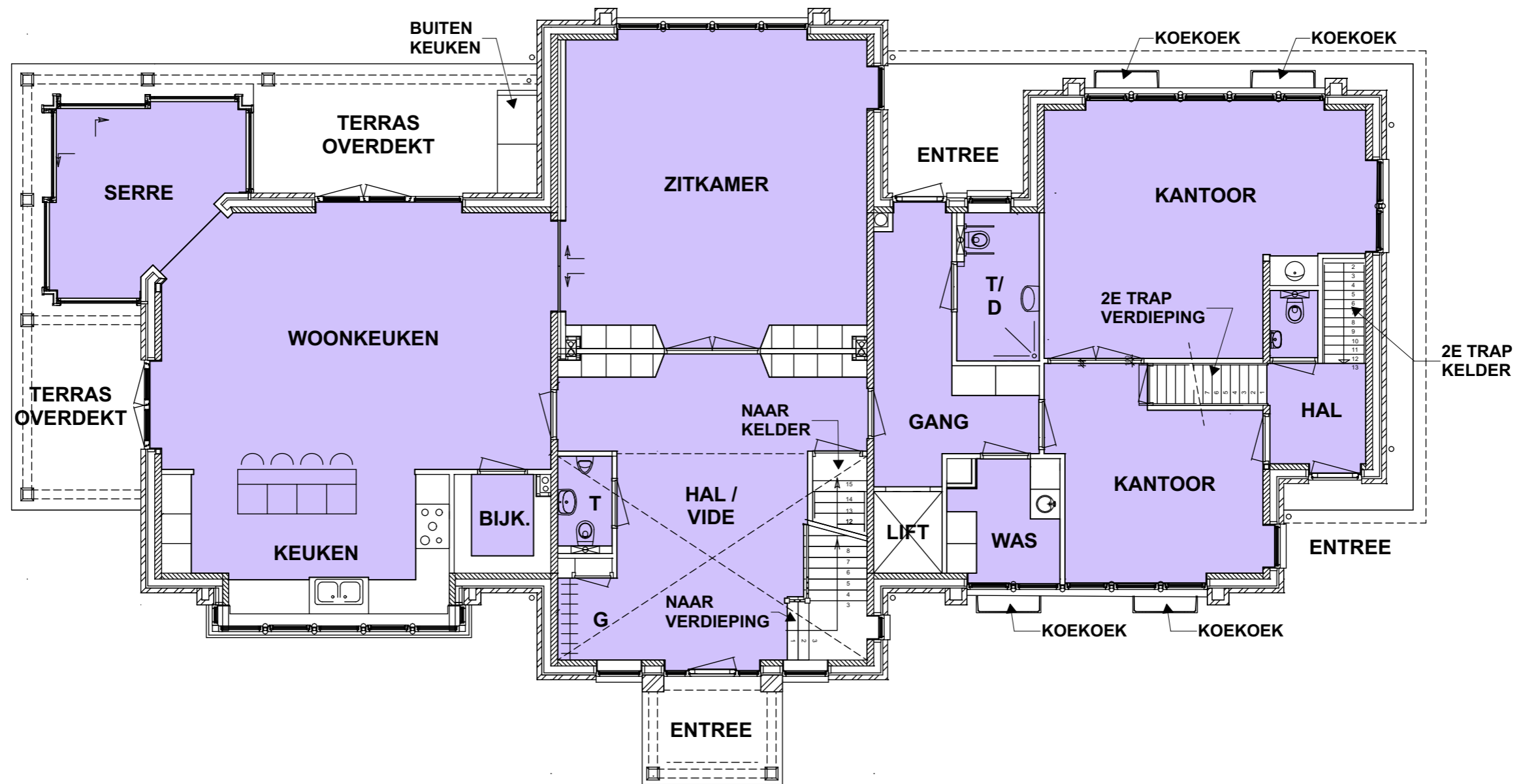
PLATTEGROND BEGANEGROND
