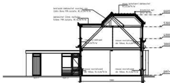
doorsnede - A-A de Wetstraat - 21 t/m. 39 oneven type H
