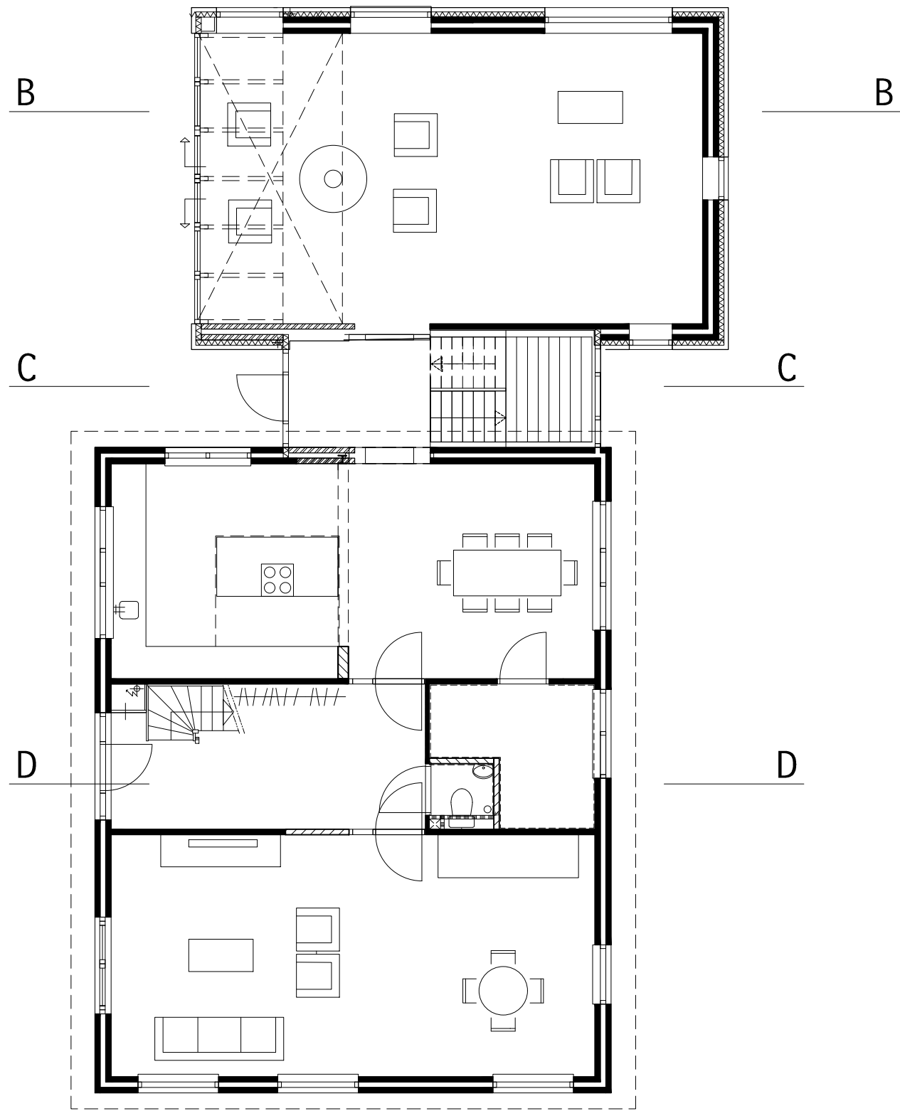
BEGANEGROND A
