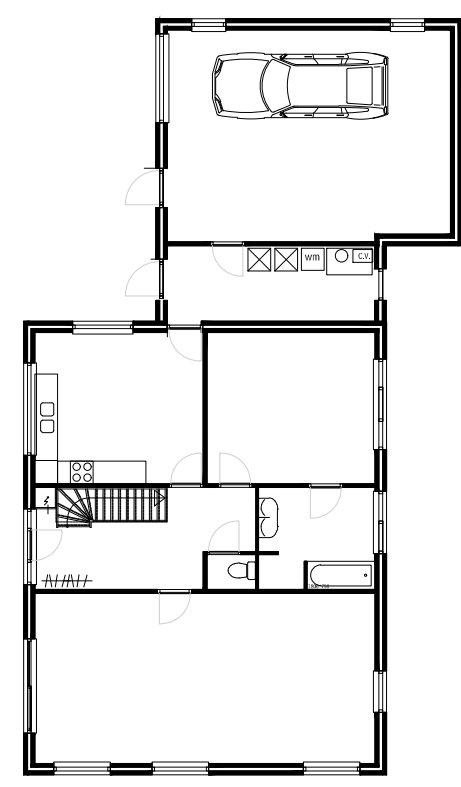
BEGANEGROND
