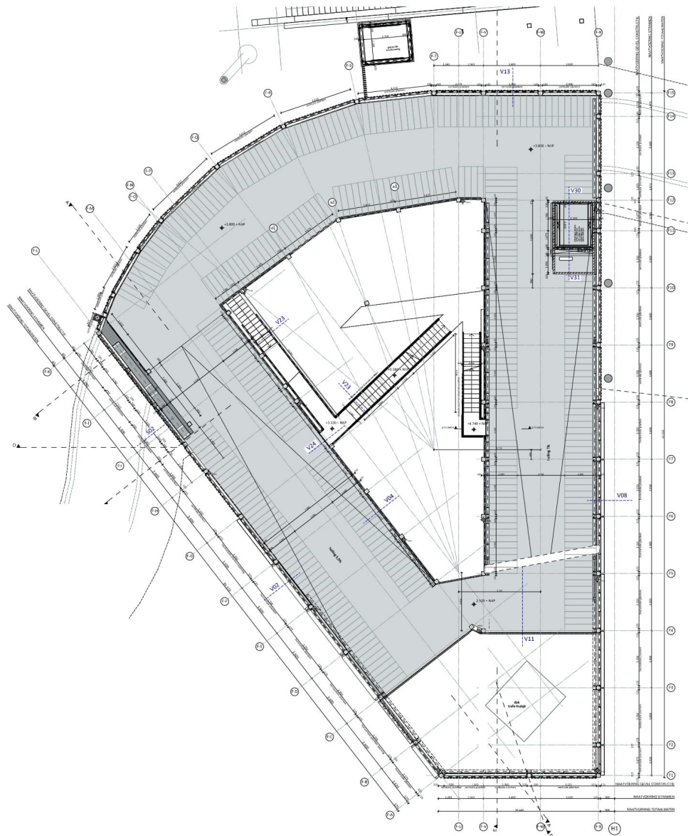
Tussenniveau +6
