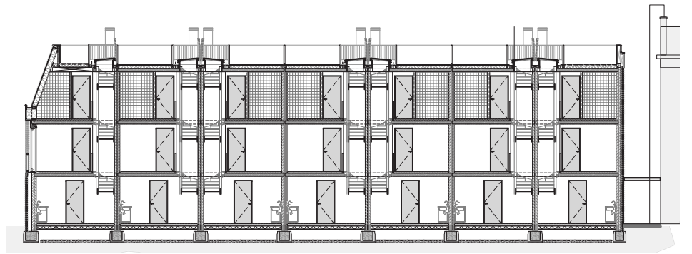
Doorsnede
