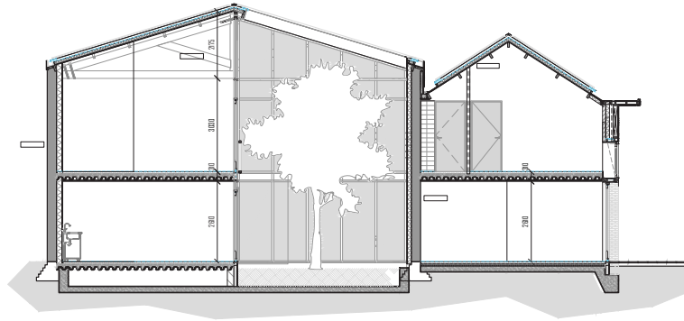
Doorsnede
