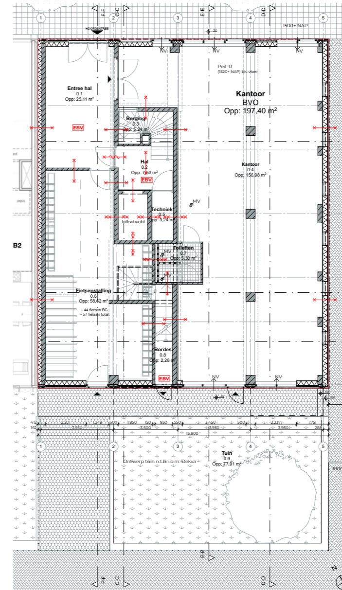
begane grond
