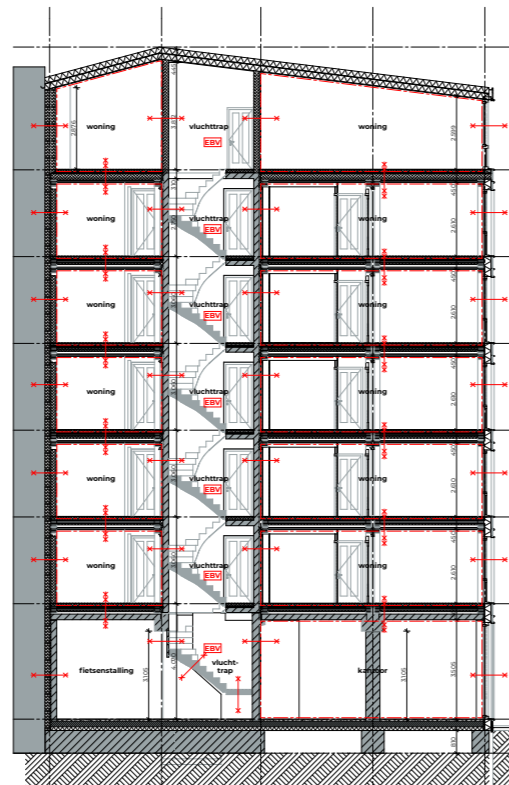
doorsnede A-A
