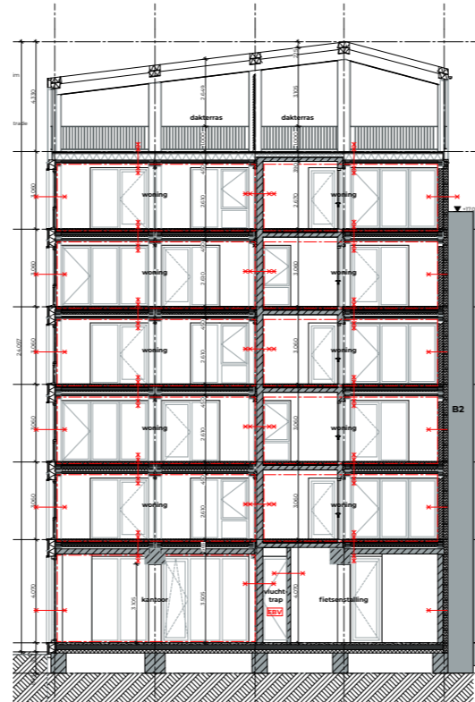
doorsnede B-B
