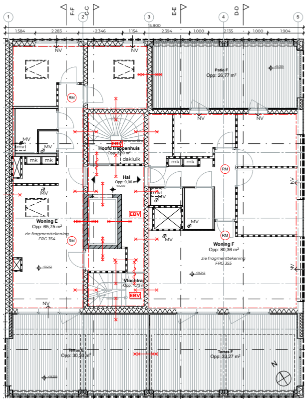
6 e verdieping
