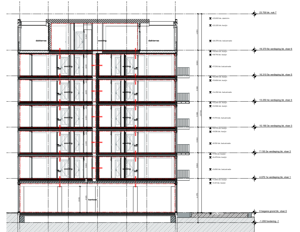
doorsnede E-E
