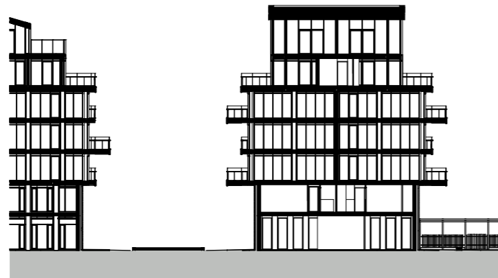
dwarsdoorsnede
