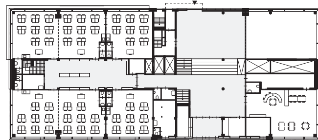
begane grond
