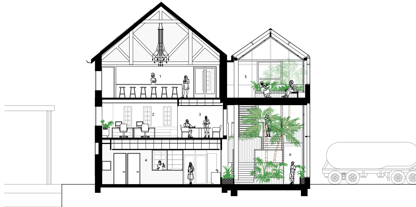
Langs- en dwarsdoorsnede gebouw
