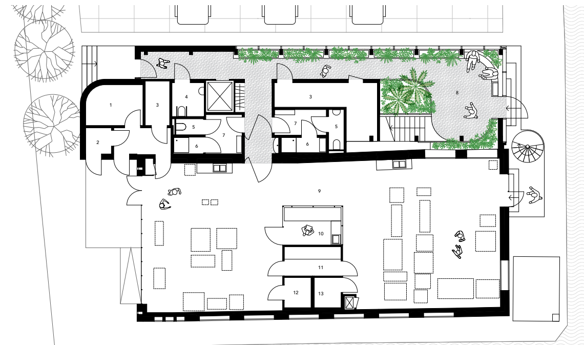
Plattegronden begane grond en 1e verdieping
