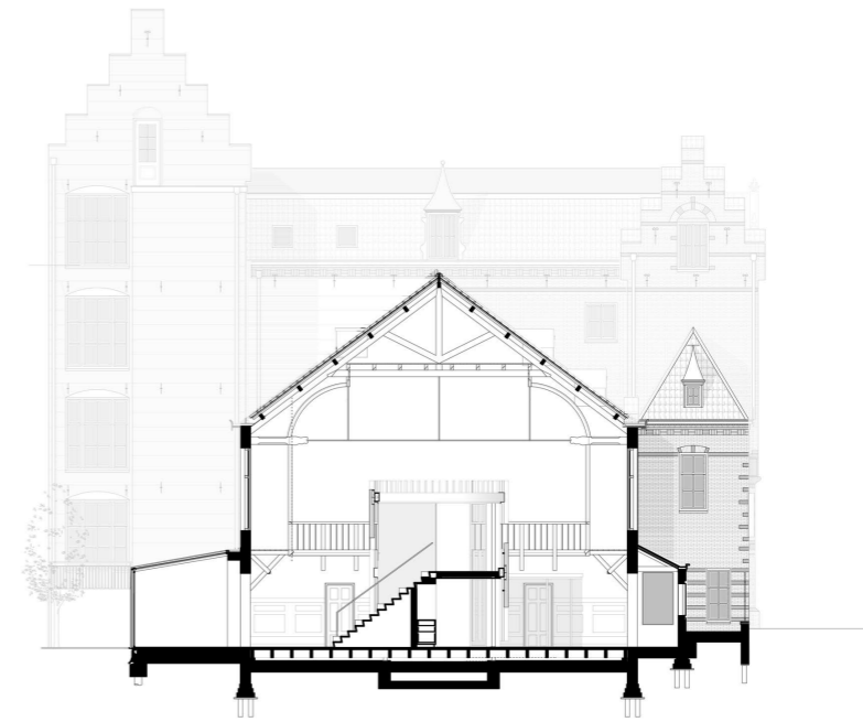
DWARSDOORSNEDE
