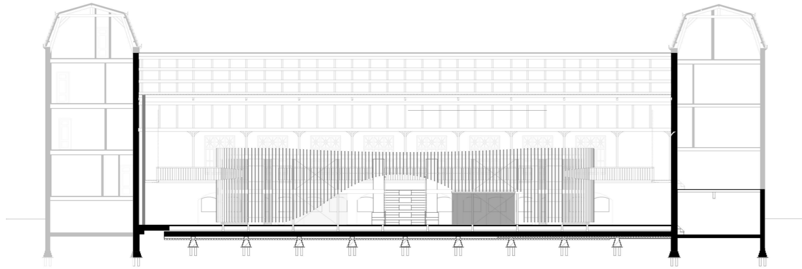
NOORD GEVEL BINNEN
