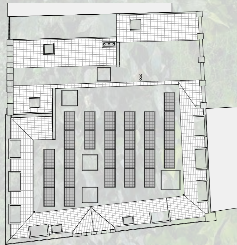
Plattegrond dak
